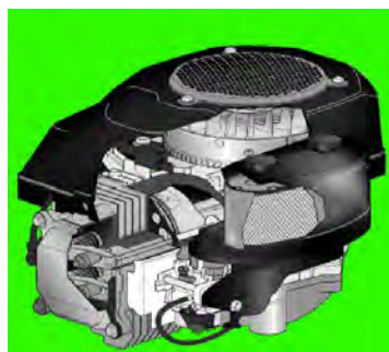
Art. GGP ITALIJA MOTOR ZA KOSA ICU GGP 160 OHV Silent SNAGA 5hp / 160 cc MAX. BROJ OBRTAJA 3000 RADILICA 22.2 X 55
