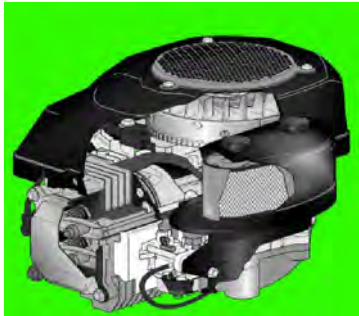
Art. GGP ITALIJA MOTOR ZA KOSA ICU GGP SV150 SNAGA 3.5 hp / 135 cc MAX. BROJ OBRTAJA 3000 RADILICA 22.2 X 55
